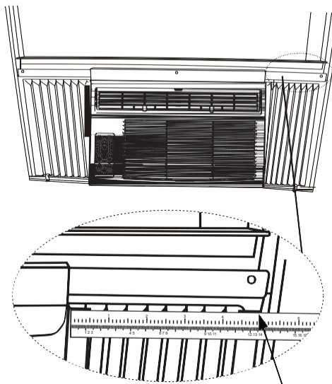
Mida el ancho interior de la cortina lateral
